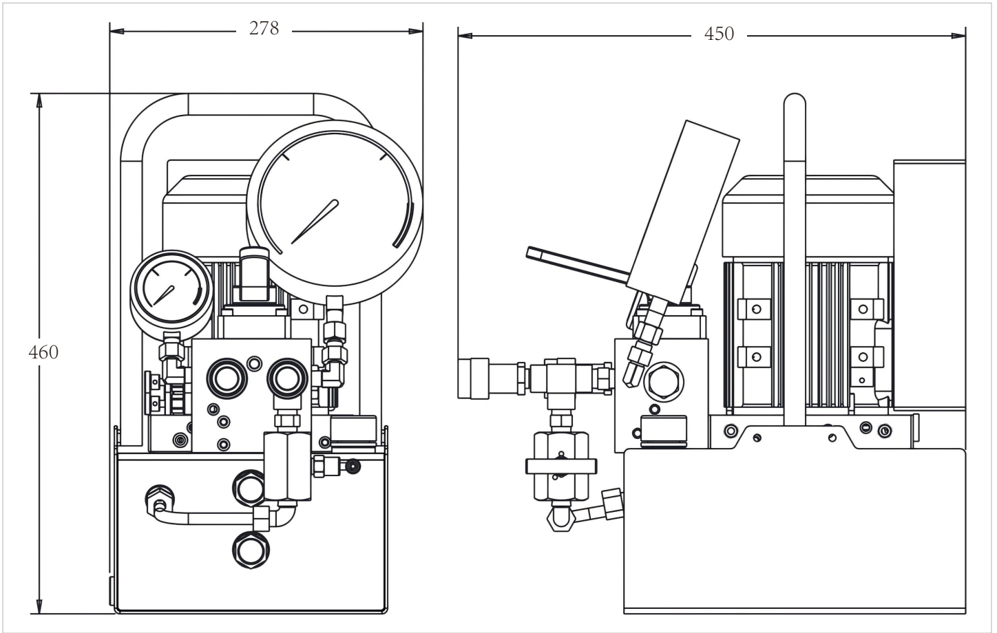
▼ HE4007MVL43-SP 外形图:
