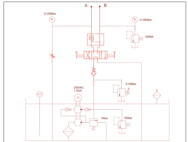
▼ 液压原理图:
